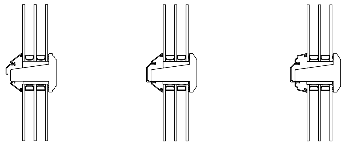
Rundad profil insida - Vinklad glaslist utsida
