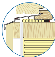
HCP tröskel
