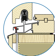
Skjuddörr tröskel
